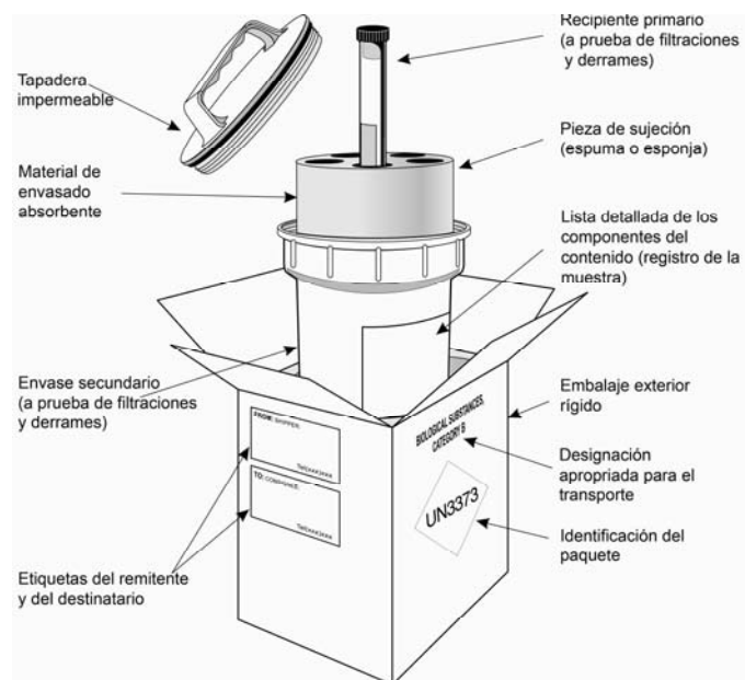
Figura 9. Ejemplo de sistema de embalaje/ensado triple para el embalaje y etiquetado de sustancias infecciosas de categoría B (por cortesía de la IATA, Montreal, Canadá)
